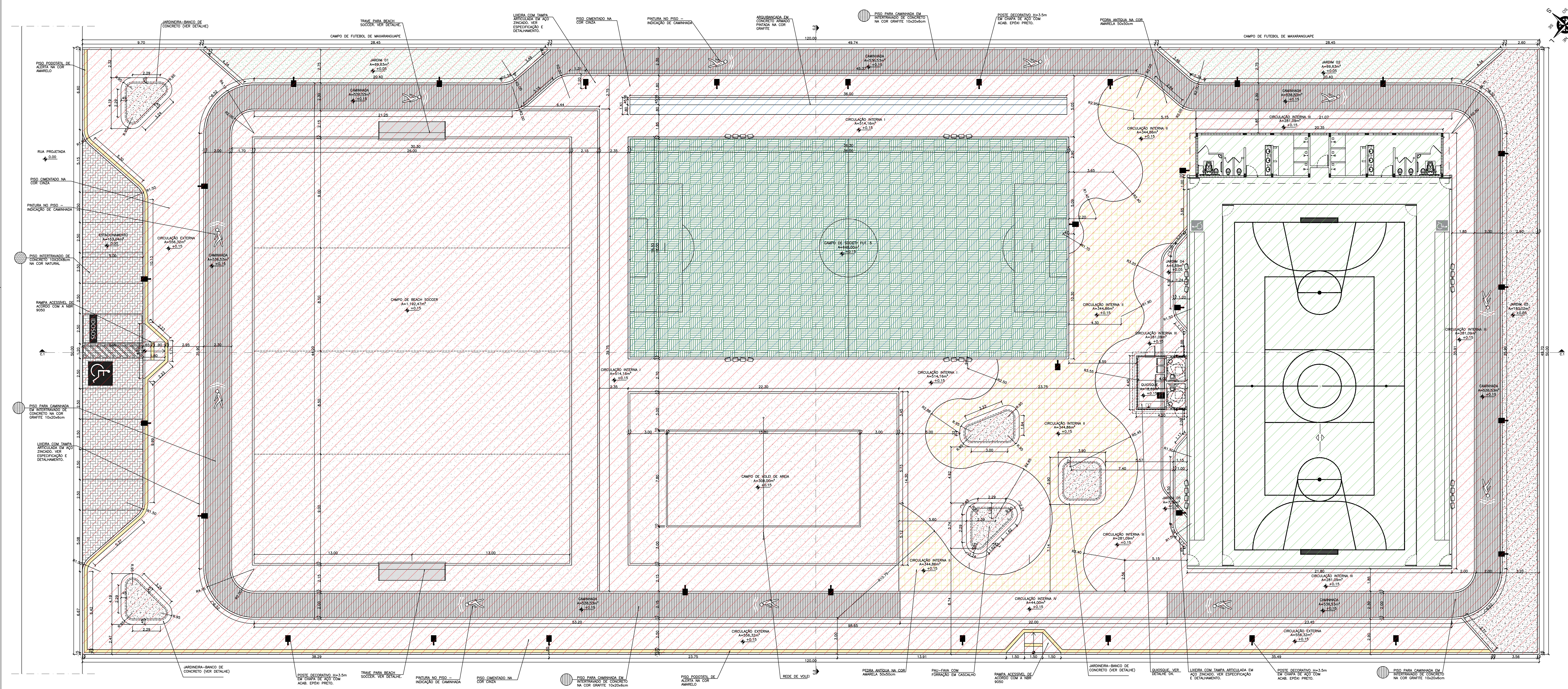
PLANTA ILUMINADA Complexo Esportivo, Maxaranguape/RN Escala: 1/125
